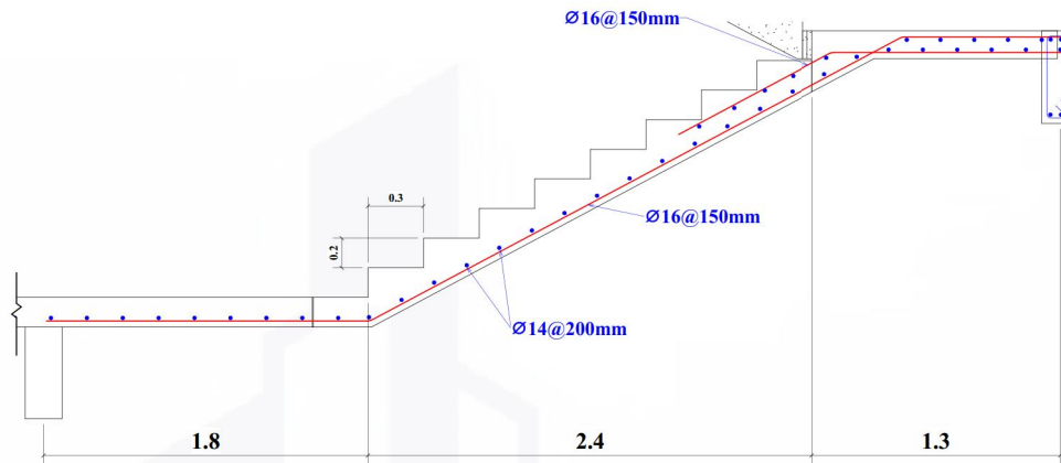
1 stair 1 : 20
