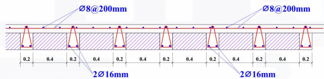
2 rib 1 : 20
