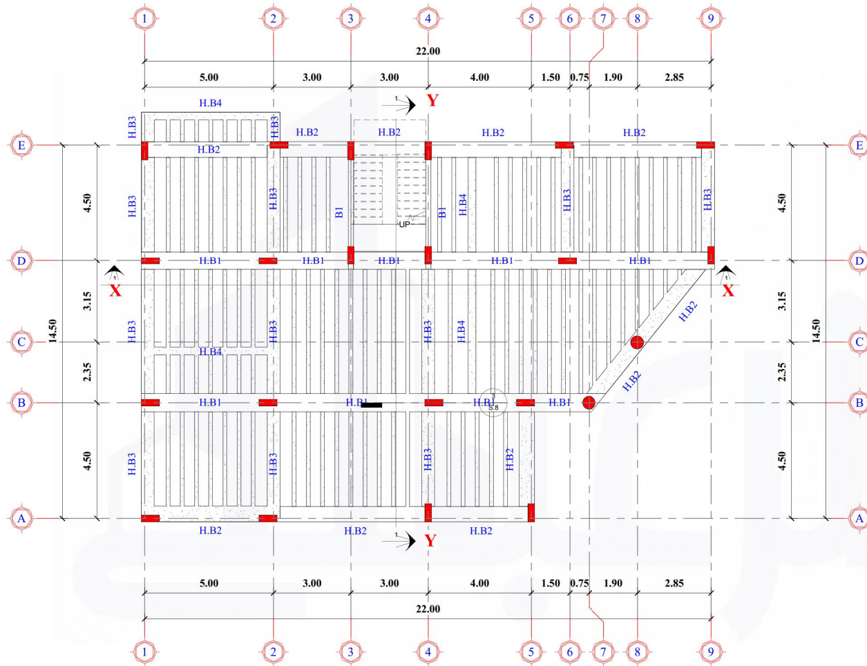
مخطط سقف البدوم 1 1 : 90
