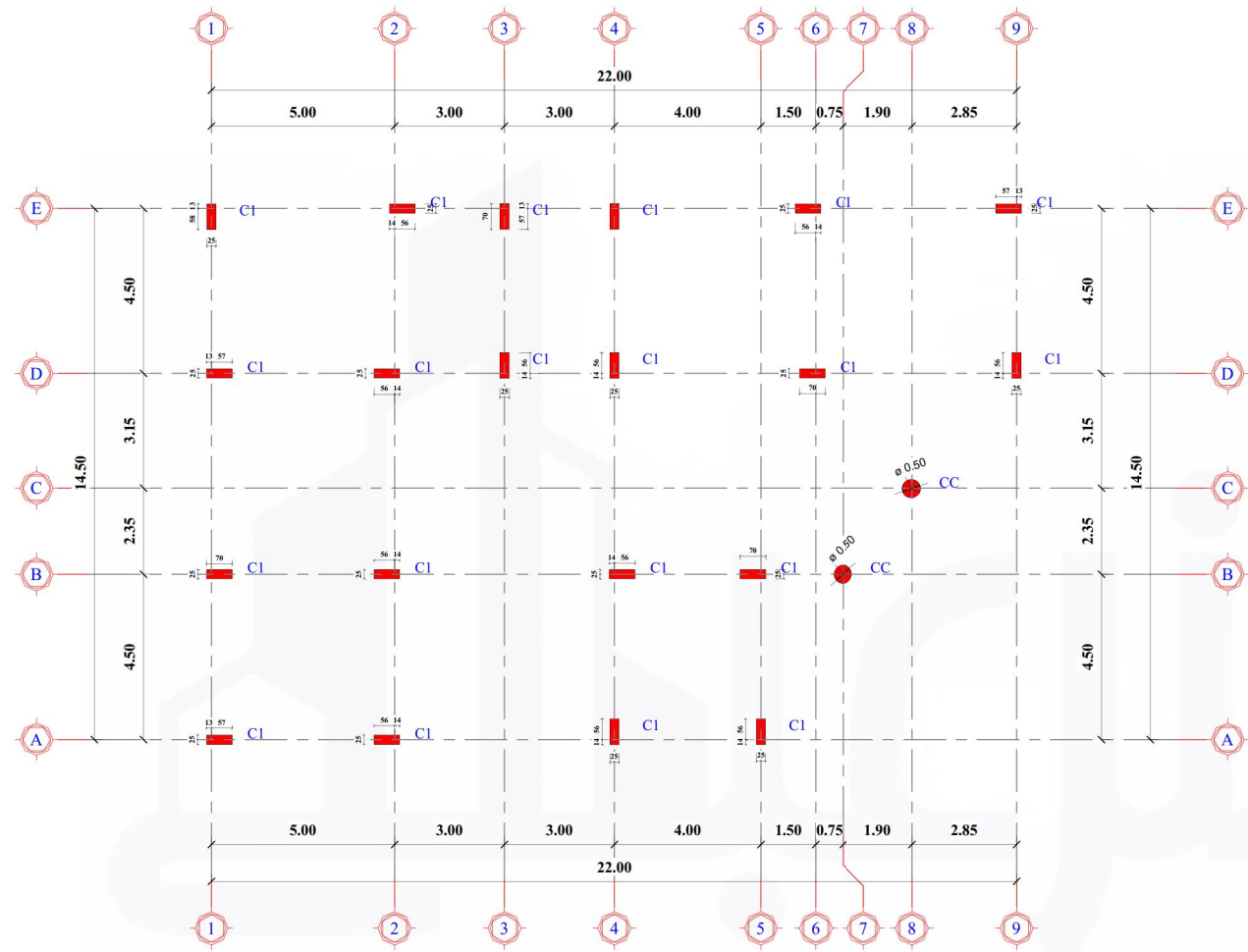
مخطط محاور الاعمدة 3 1 : 90
