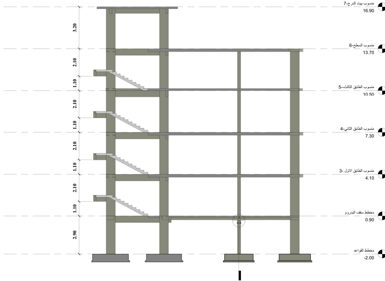
1 Section Y-Y 1 : 80
